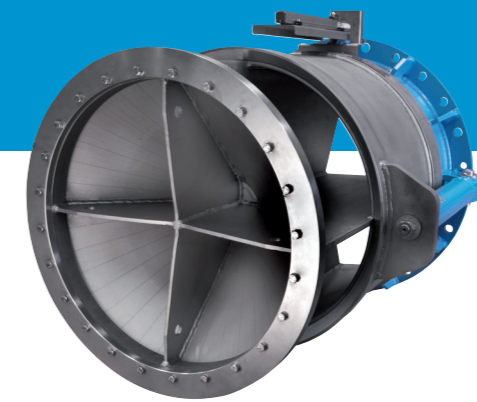
CH Válvula de chorro hueco. Fixed cone valve. Kegelstrahlschieber.
