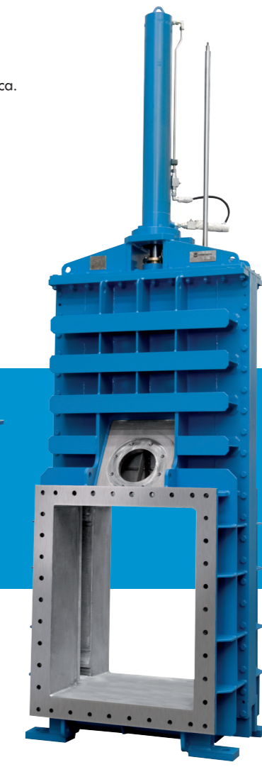
BU Compuerta "Bureau". Bonneted gate. Ablass-, Regel- und Absperrschieber in Rechteckform.
