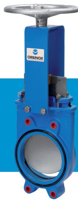
EB V.G. bidireccional. Bidirectional K.G.V. Zweiseitig dichtender Stoffschieber.
